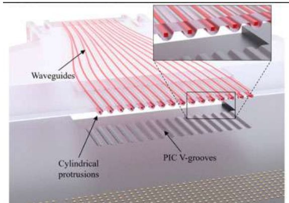
Edge Coupling FAU
