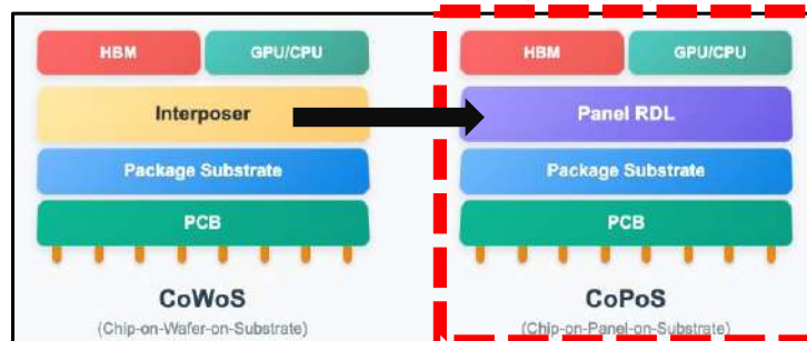
CoWoS、CoPoS技術示意圖
