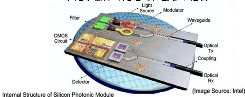
矽光子晶片之光電元件整合示意圖
