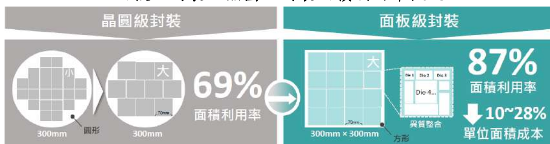
面板級封裝、晶圓級封裝面積利用率概況
